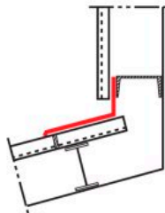
11.- Coronación en albardilla
