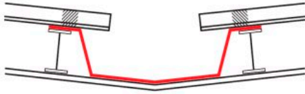
1.- Canalón central
