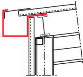
3.- Canalón lateral exterior
