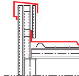
10.- Coronación en alto de pendiente
