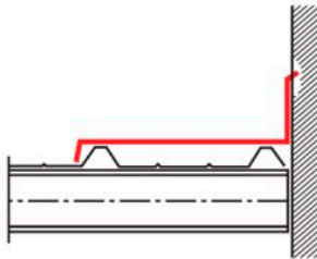
9.- Alto de pendiente a fachada
