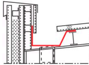
4.- Canalón de diente de sierra
