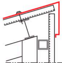
12.- Coronación en lateral de pendiente
