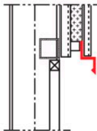
19.- Superior de ventana
